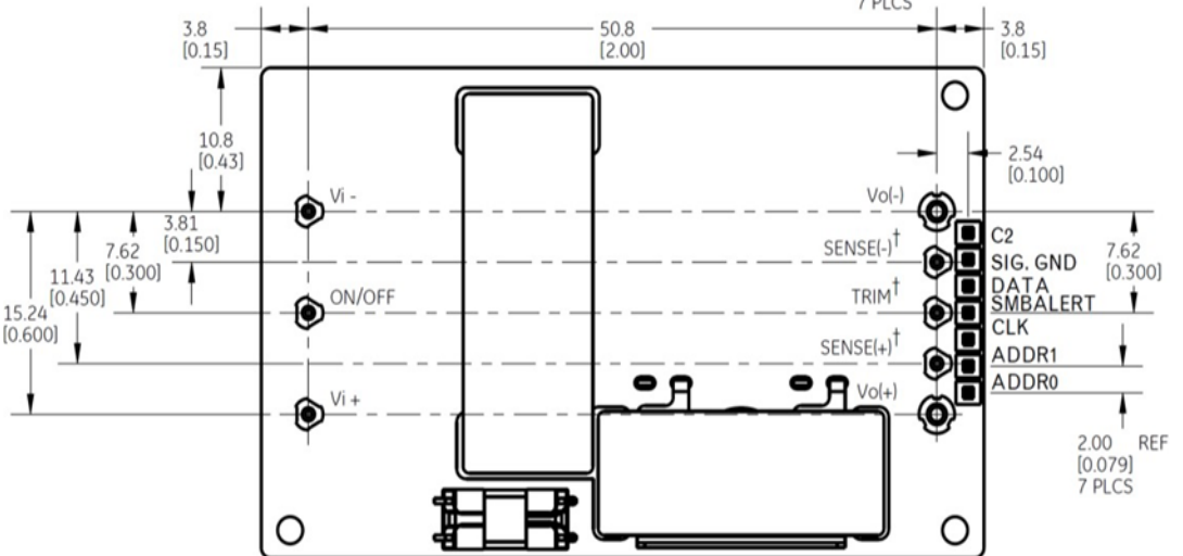
BOTTOM VIEW***
