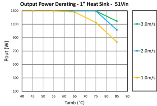
(b) V_{IN}=51V
